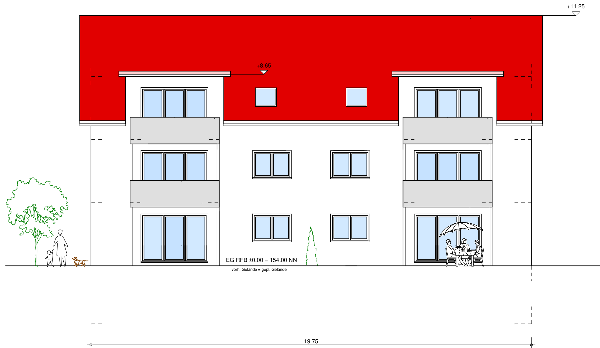
Ansicht Süd-West
