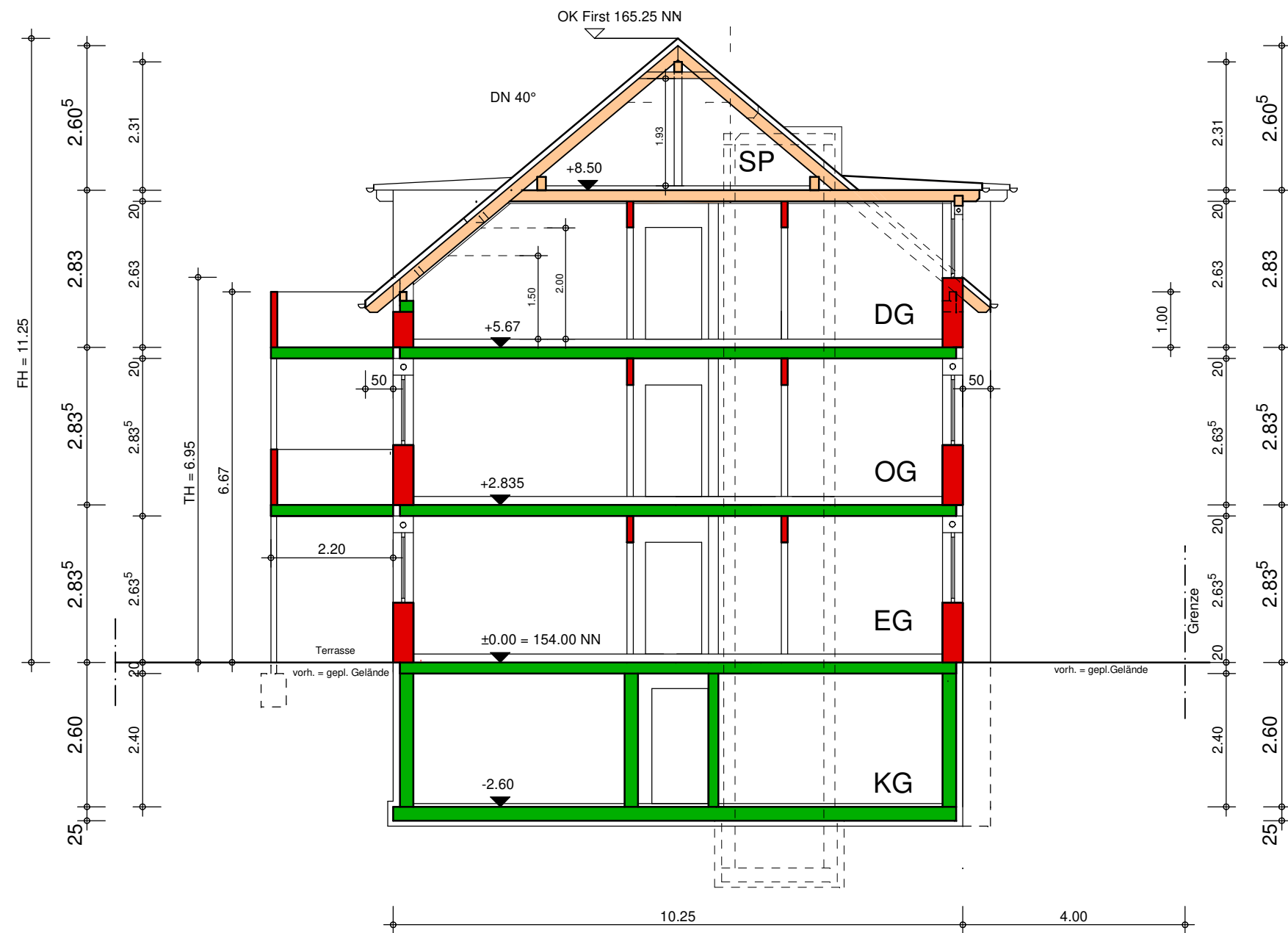
SCHNITT A-A
